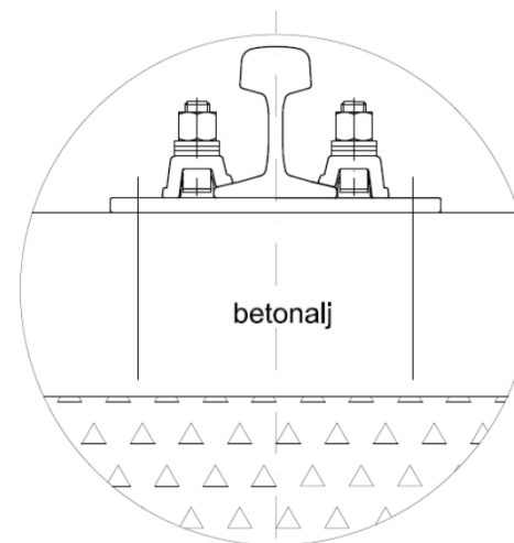
Zúzottkő ágyazatú pálya
